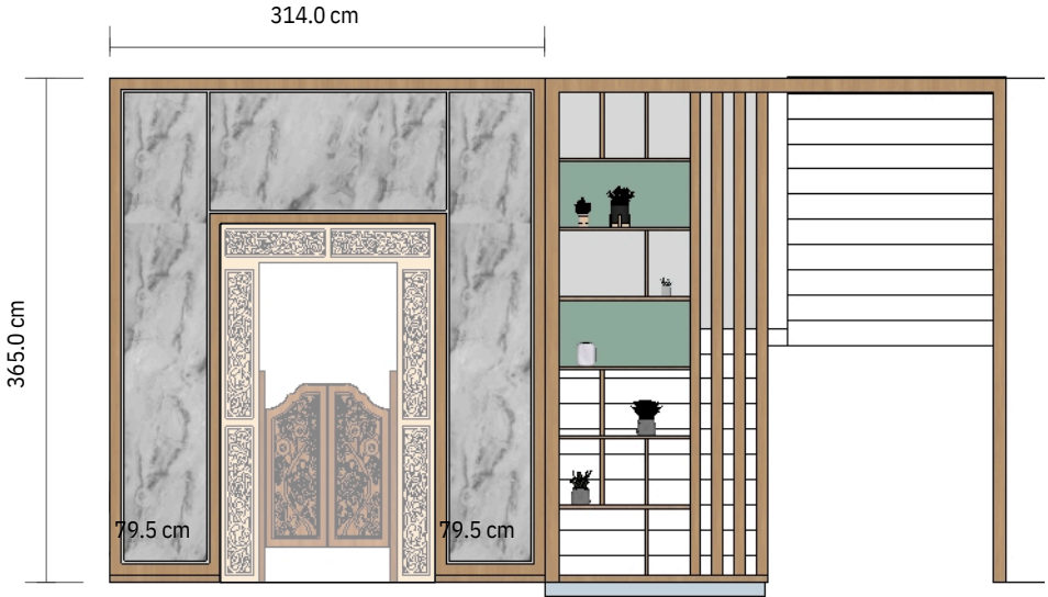
A :: Tampak Depan 001 scale: 1:60
