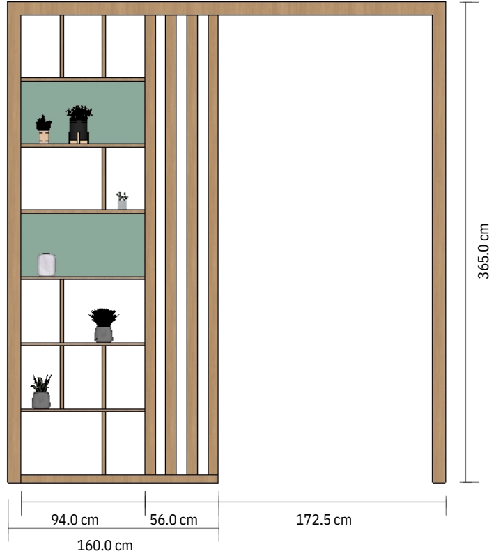
A :: Tampak Depan 001 scale: 1:40
