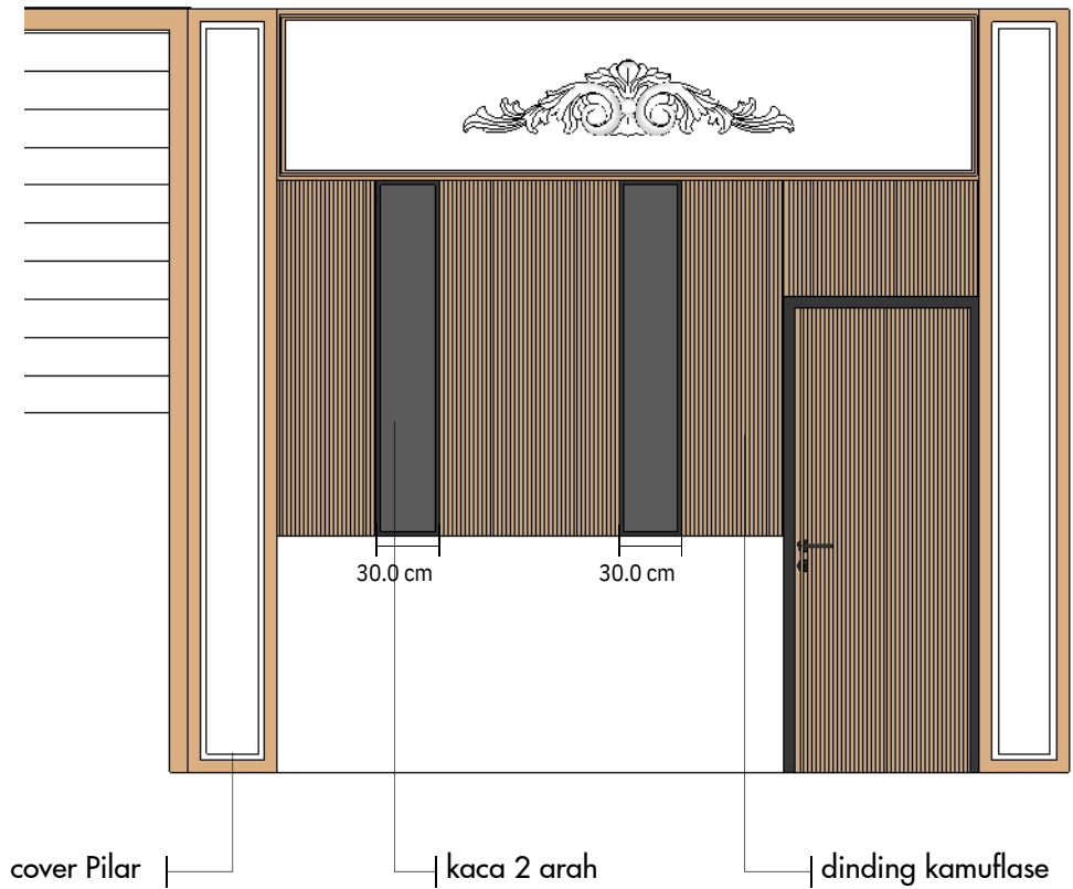
A :: Tampak Depan 001 scale: 1:40
