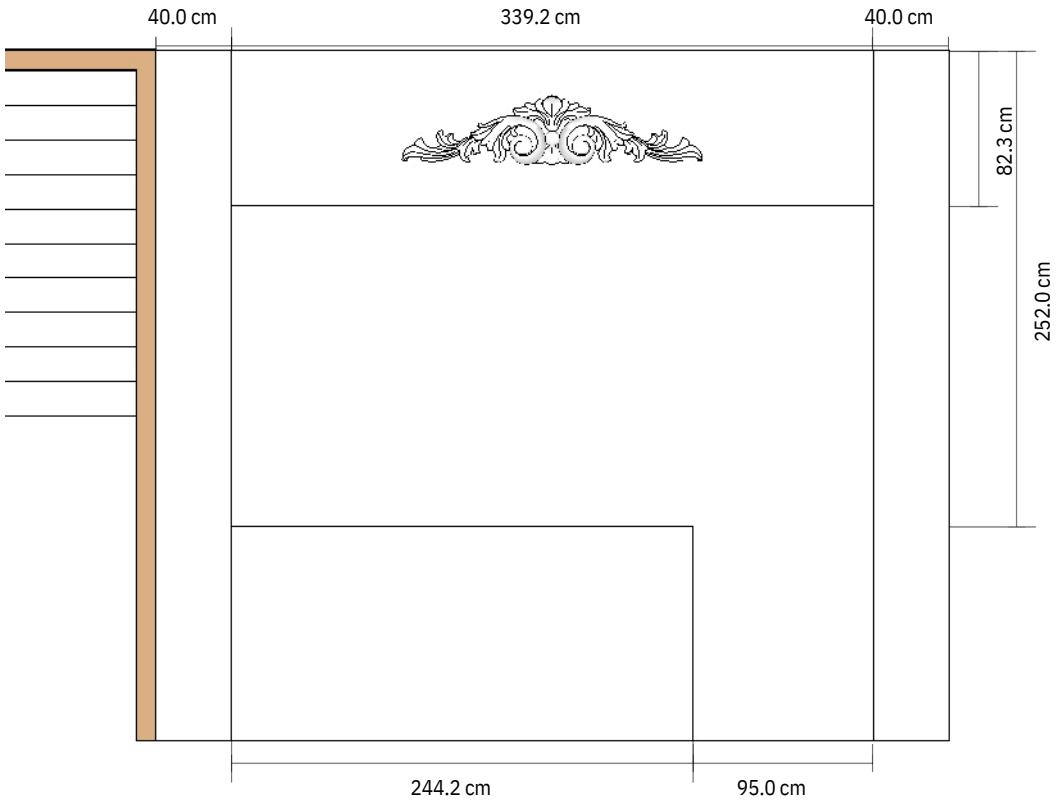
A :: Tampak Depan 001 scale: 1:40
