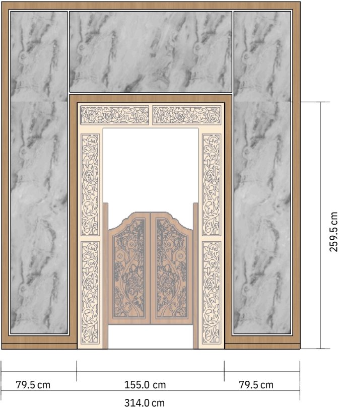
A :: Tampak Depan 001 scale: 1:40
