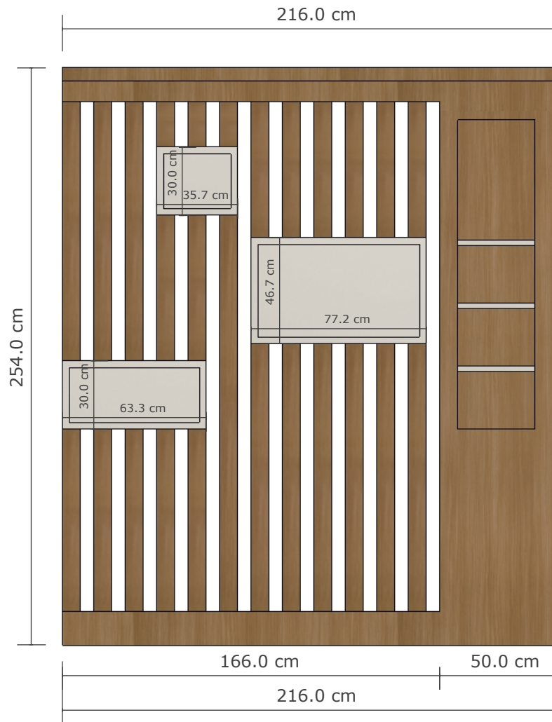
A :: PARTISI 001 tampak depan
