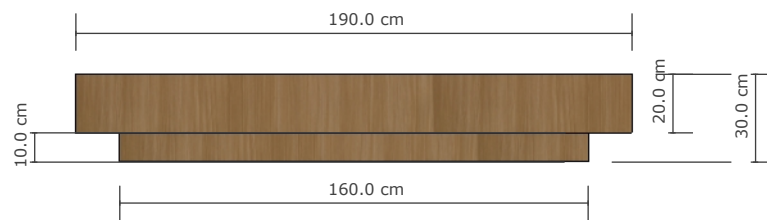
A :: DIVAN 002 tampak depan
